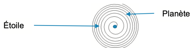
FIGURE 7 – Représentation fictive de la trajectoire d'une planète qui « tomberait » sur son étoile
