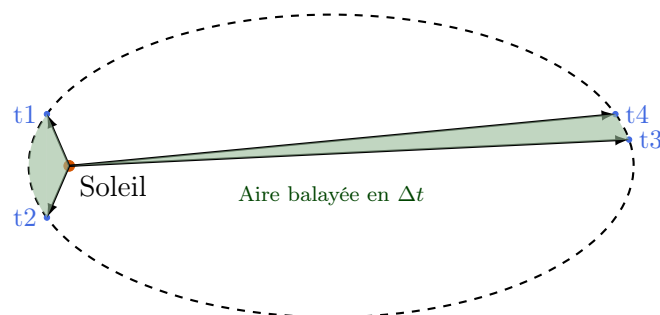
FIGURE 5 – Schéma illustrant la loi des aires
