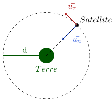
FIGURE 3 – Satellite en orbite circulaire autour de la Terre
