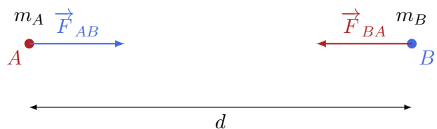
FIGURE 2 – Force gravitationnelle entre deux masses
