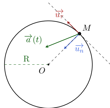
FIGURE 1 – Repère de Frenet
