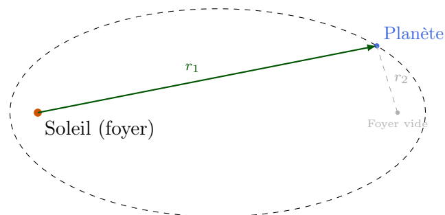
FIGURE 4 – Trajectoire elliptique, Soleil en foyer
